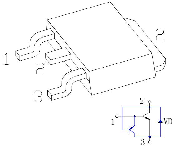
1 基极(B) 2 集电极(C) 3 发射极(E)
